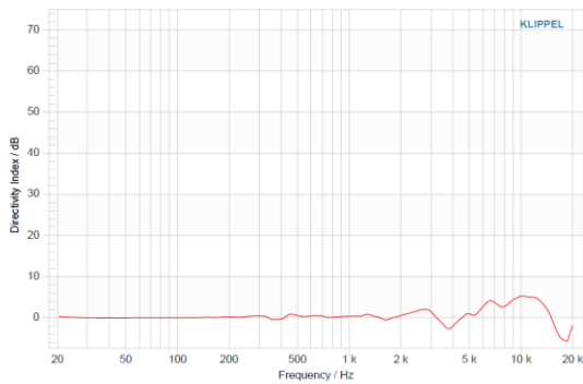
・指向性指数-周波数 DIRECTIVITY INDEX VS FREQUENCY
