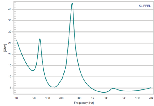
・インピーダンス - 周波数 IMPEDANCE VS FREQUENCY
