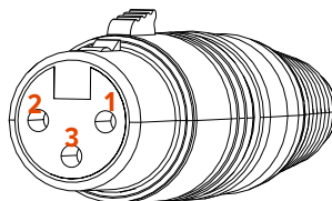
XLR 端子メス バランス配線
