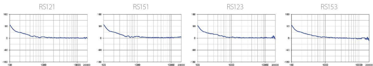
放射角
