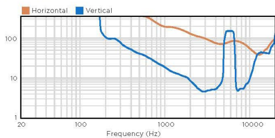
ビーム幅
