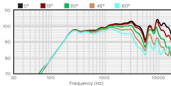
垂直軸外ダウン応答
