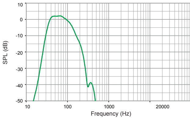
周波数特性：プロセッシング済みバイアンプの場合 LF= 緑
