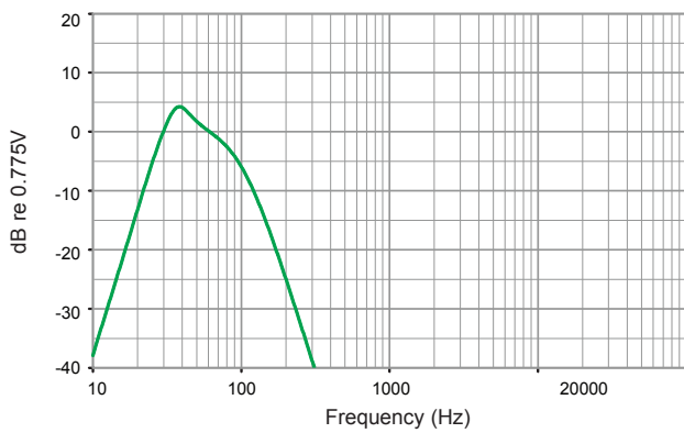
周波数特性：デジタルシグナルプロセッサー LF= 緑
