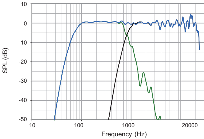
周波数特性：プロセッシング済み、バイアンプの場合 LF = 緑 HF = 黒 全体 = 青
