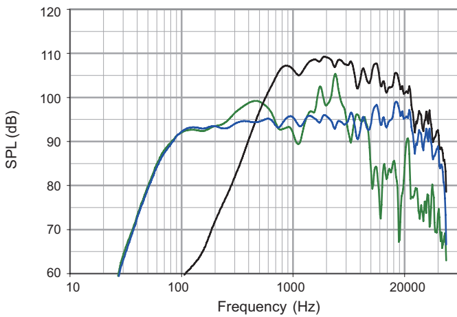
周波数特性：プロセッシングしていない場合 LF = 緑 HF = 黒 全体 = 青
