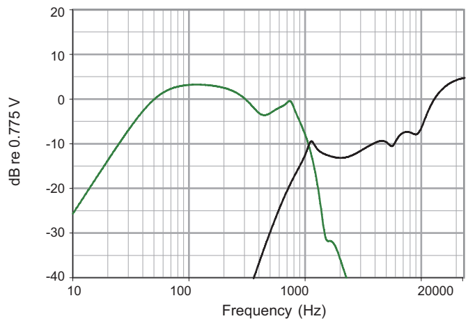
周波数特性：デジタルシグナルプロセッサ LF = 緑 HF = 黒
