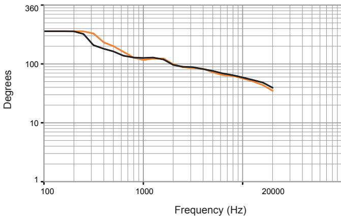
放射幅 水平 = 橙 垂直 = 黒
