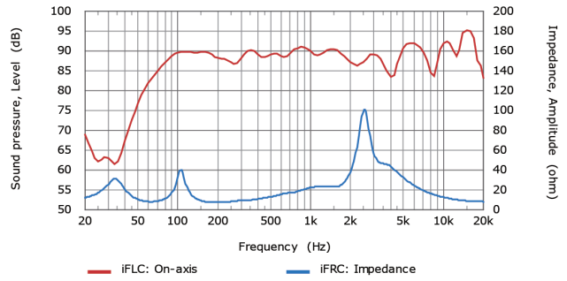
インピーダンス / 周波数特性
