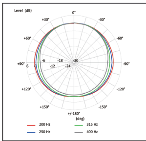
水平指向特性
